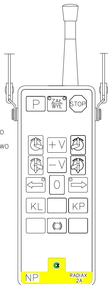
NADAJNIK POMOCNIKA
