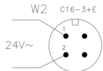
ZŁĄCZE SZUFLADOWE 871050
