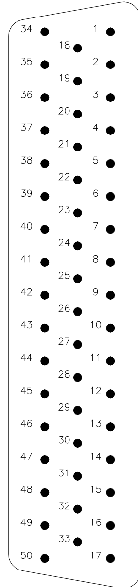
ZŁĄCZE SZUFLADOWE 871050
